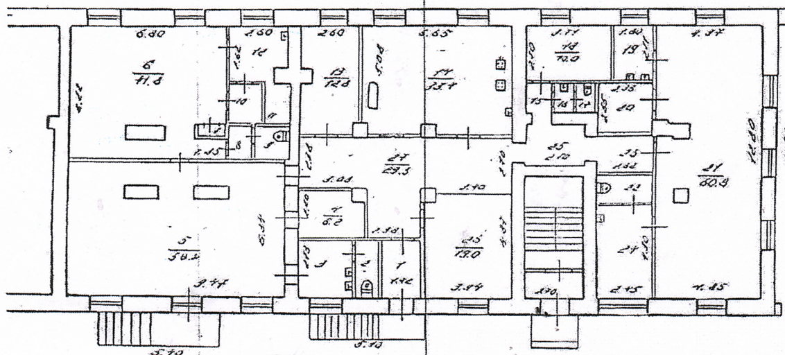
План 1 этажа
